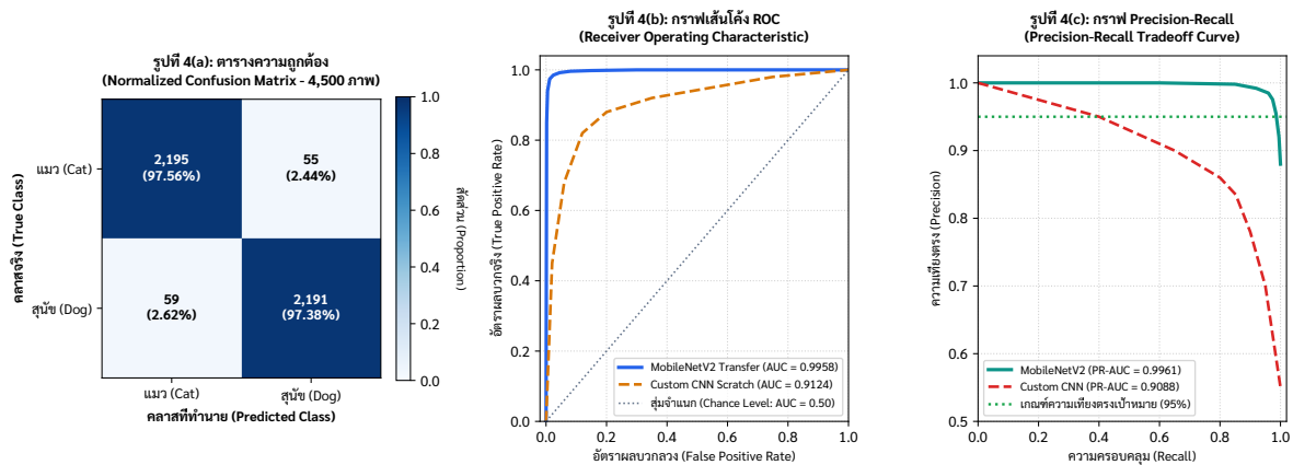
รูปที่ 4: การวินิจฉัยผลการจำแนกเชิงลึก: (a) Normalized Confusion Matrix (b) กราฟเส้นโค้ง ROC (AUC = 0.9958) (c) กราฟ Precision-Recall Tradeoff (PR-AUC = 0.9961)
