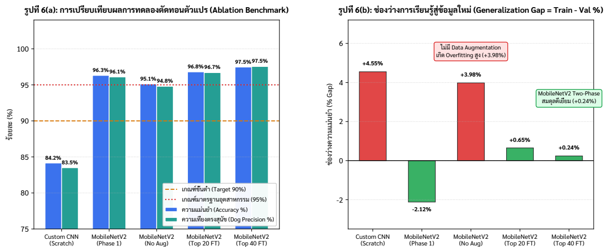
รูปที่ 6: การทดลองตัดทอนตัวแปร (Ablation Study): (a) เปรียบเทียบความแม่นยำและความเที่ยงตรงของโมเดล 5 รูปแบบ (b) การวิเคราะห์ Generalization Gap ( |Train - Val| %)
