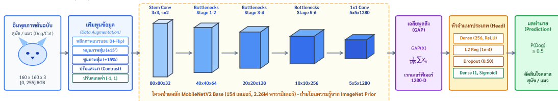
รูปที่ 2(a): ผังท่อส่งข้อมูลเทนเซอร์และการเรียนรู้แบบถ่ายโอน (End-to-End Transfer Learning & Tensor Pipeline)
