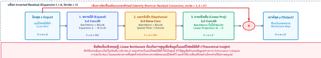
รูปที่ 2(b): โครงสร้างจุลภาค Inverted Residual Block พร้อมคอขวดเชิงเส้น (Micro-Architecture)
